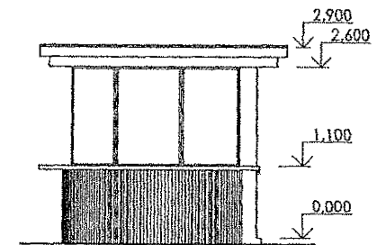
Фасад М 1:50
