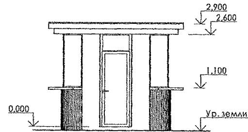
Фасад М 1:50
