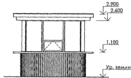
Фасад М 1:50
