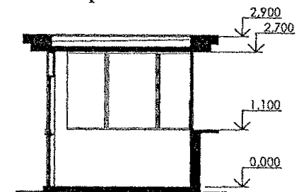
Разрез М 1:50
